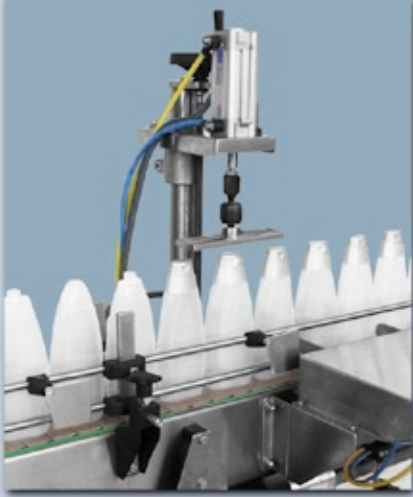
Çakpa Kapak Kapama Ünitesi Pushing Head
